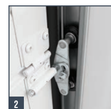
2 Galets double pour un fonctionnement souple et silencieux
