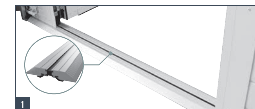
1 Seuil plat en aluminium (normes PMR) à rupture de pont thermique + 2 joints EPDM
