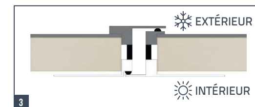
3 Profils à rupture de pont thermique
